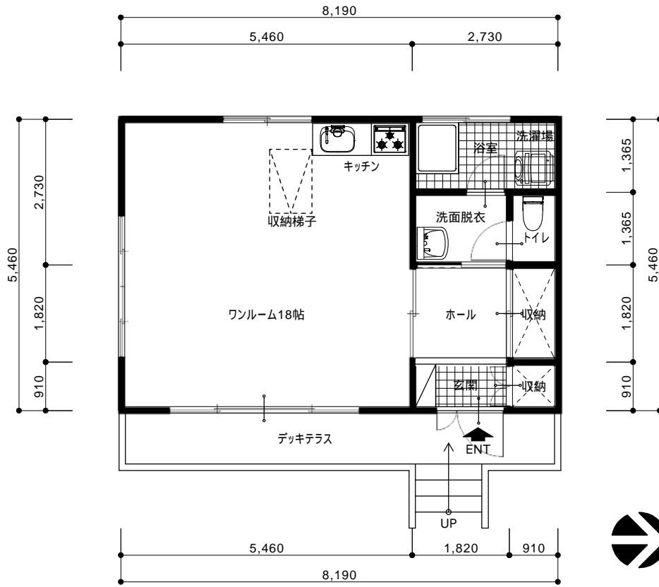
1階 平面図 1 : 100
