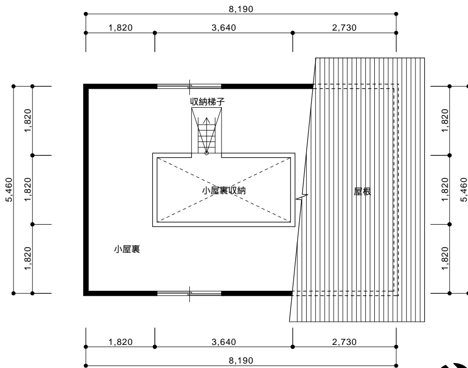
小屋裏 平面図 1 : 100
